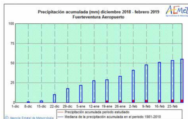
erteventura Aeropuerto. Precipitación (mm)
